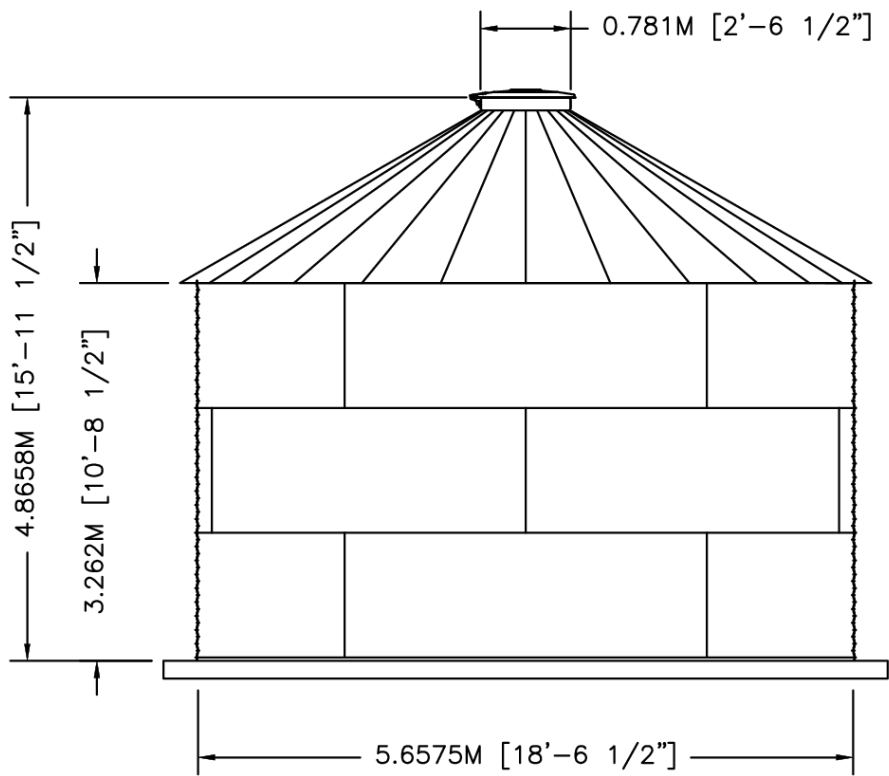
ELEVATION
